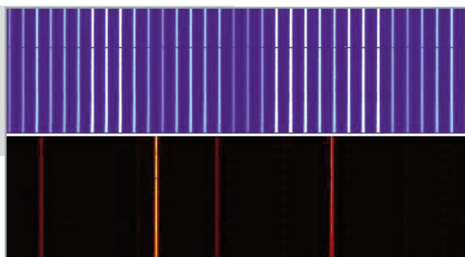
Comparación del espectro del peine de luz (arriba) con el de una lámpara de neón que muestra las ventajas del primero al producir más líneas de emisión y más regulares que la lámpara convencional. Izda: telescopio de 3,5 metros del observatorio de Calar Alto.
