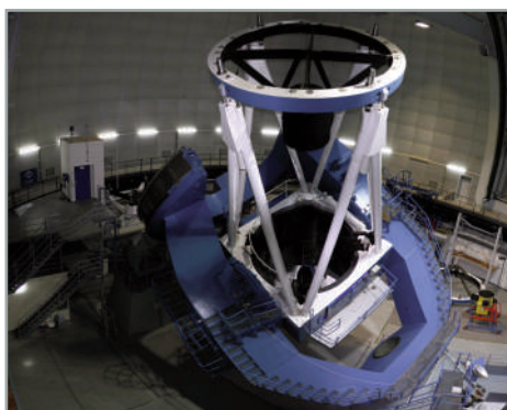
Comparación del espectro del peine de luz (arriba) con el de una lámpara de neón que muestra las ventajas del primero al producir más líneas de emisión y más regulares que la lámpara convencional. Izda: telescopio de 3,5 metros del observatorio de Calar Alto.
